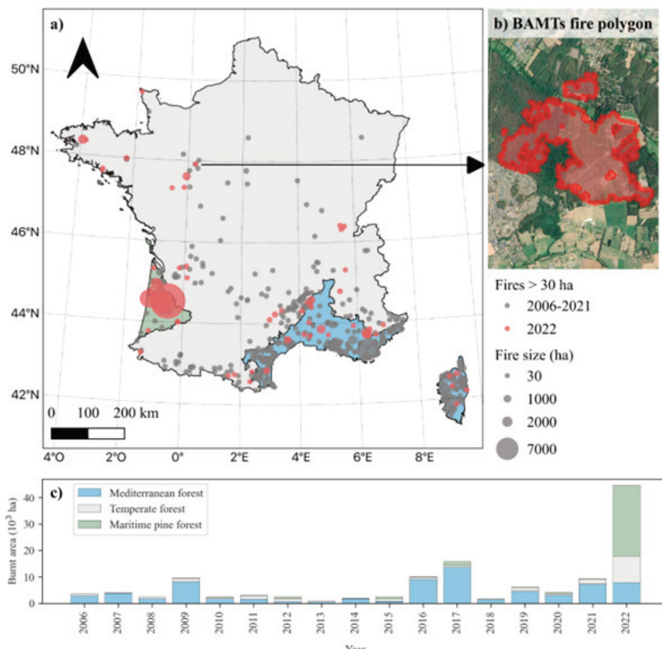
Figure 9. Observations par satellite des surfaces brûlées en France en 2022, montrant l'augmentation inédite en 2022 des feux dans les Landes (en vert) et diverses forêts tempérées en Bretagne, Pays de la Loire et Jura (en gris). Source : Vallet et al. 2023.
