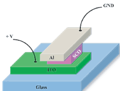
Elaboration d'une jonction composée d'une couche d'aluminium, une couche de 30 nm d'un matériau moléculaire bistable, d'une couche d'un conducteur transparent (ITO) et d'un substrat en verre
