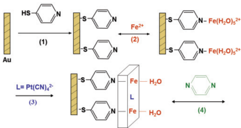
Protocole de synthèse chimique séquentiel "couche par couche" permettant d'obtenir des couches minces électriquement bistables
