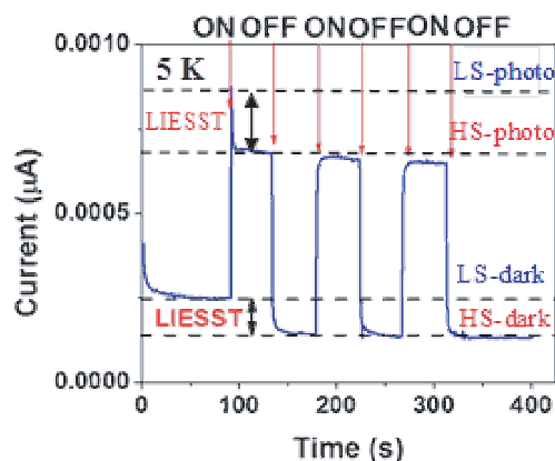
Mesure d'un photo-courant au travers cette jonction montrant des valeurs différentes selon que le matériau est dans son état haut spin ( S=2 ) ou bas spin ( S=0 ). La valeur du photo-courant est donc dépendante de l'état de spin du matériau, conduisant à un effet de type spintronique moléculaire.
