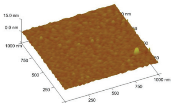
Image de microscopie à force atomique d'une couche mince obtenue avec une rugosité moyenne sub-nanométrique (de 7 Angströms)
