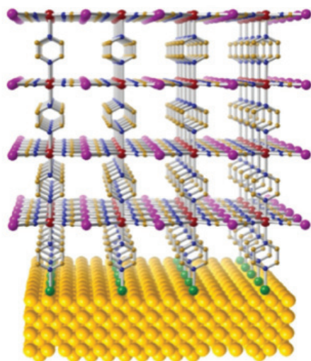
Schémas de fixation (fonctionnalisation) d'un matériau bistable sur une couche d'or via une liaison Or-Soufre
