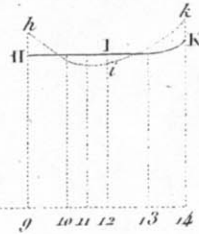
B de obscure du 3 e ordre.
