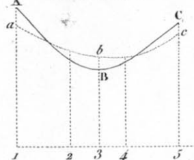
Bande obscure extérieure du 1 er ordre.
