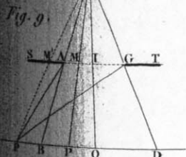
Bande obscure extérieure du 1 er ordre
