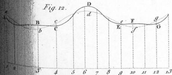
Bande obscure extérieure du 1 er ordre
